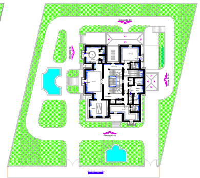
2º Andar A = 260,79 m 2
