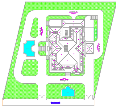
Implantação e Cobertura
